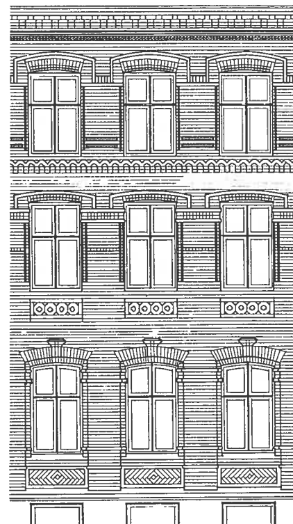
Nørregade 17, bygget 1895. Opmålt af Esbjerg Museum 1978 før nedrivningen. 2 fag af facaden er genskabt i Esbjerggudstillingen.
